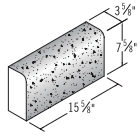
4x8x16 1F, 1T SBN*
