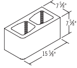
8x8x16 SBN
