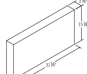
4x16x32 Solid
