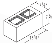
8x8x16 Korfil Insulated*
