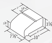
10x4x8 Sill
