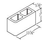
6x8x14 SBN
