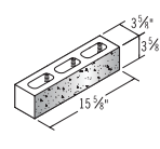
4x4x16 1F HH*
