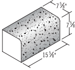
8x8x16 1F, 1T SBN*
