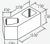
8x8x16 135° Corner Y Block
