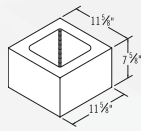
12x8x12
