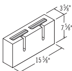
4x8x16 Acousta-Wal
