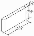
15/8x8x16
