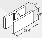
8x8x16
