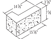
4x8x16 GFE w/ 74° Return
